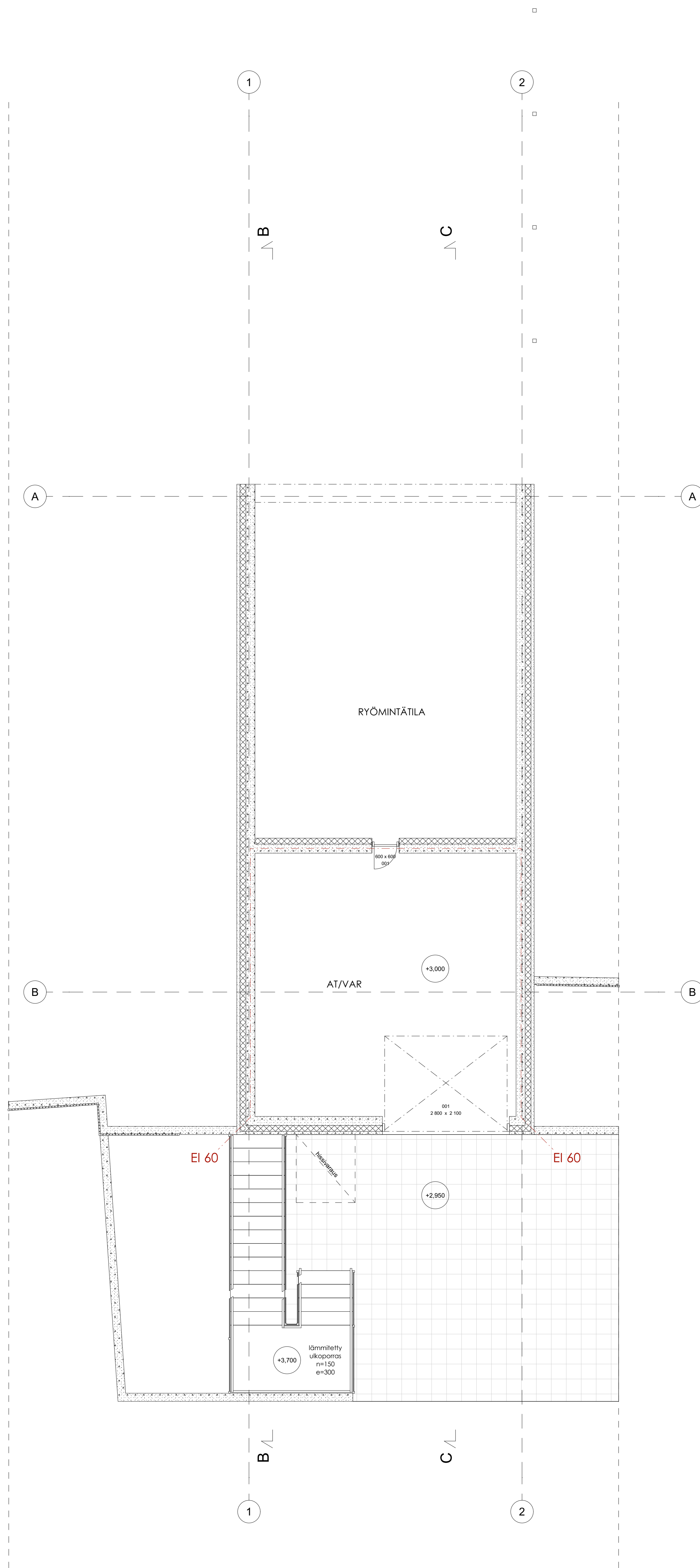
RAK. 3 KELLARI / AUTOTALLI
